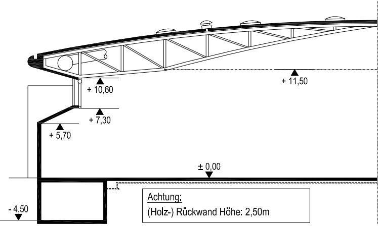
SCHNITT
